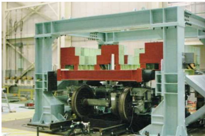
実物大台車加振試験による地震時の台車挙動の解析 Experimental analysis of seismic vehicle motion on a large-scale shaking table
